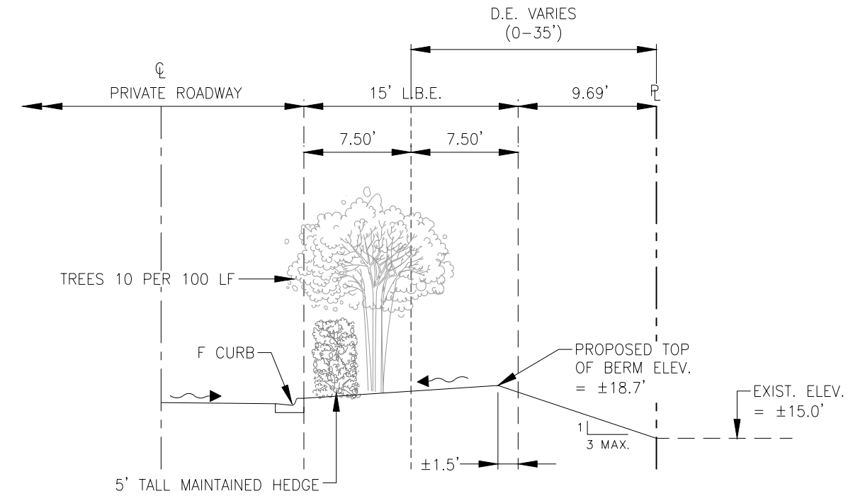
CROSS SECTION B N.T.S.
